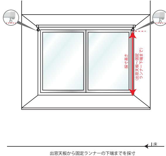
【出窓の場合】
