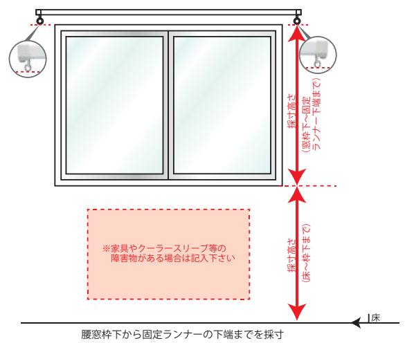
【腰窓の場合】
